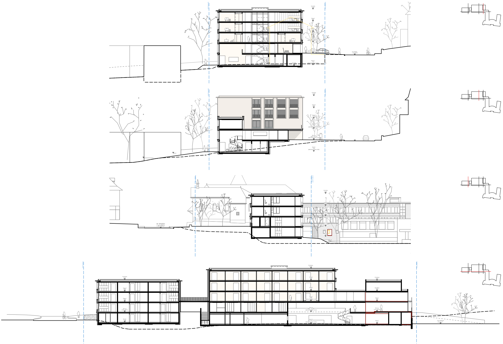
Coupes générales
